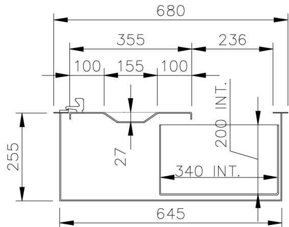
longitudinal section
